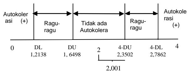
Gambar 2. Hasil Uji Autokolerasi
